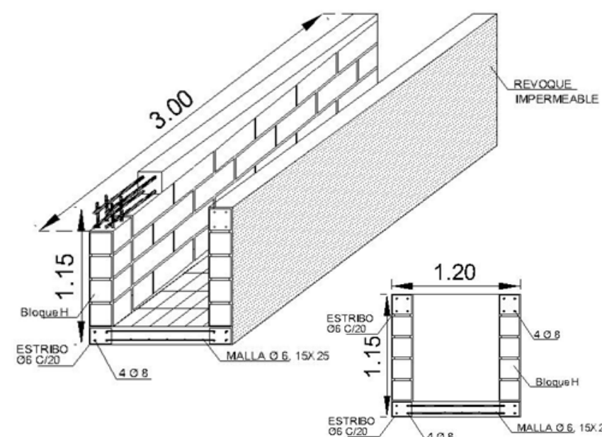
Detalle 1 y 2 del canal de desagüe para el barrio El Salado.
